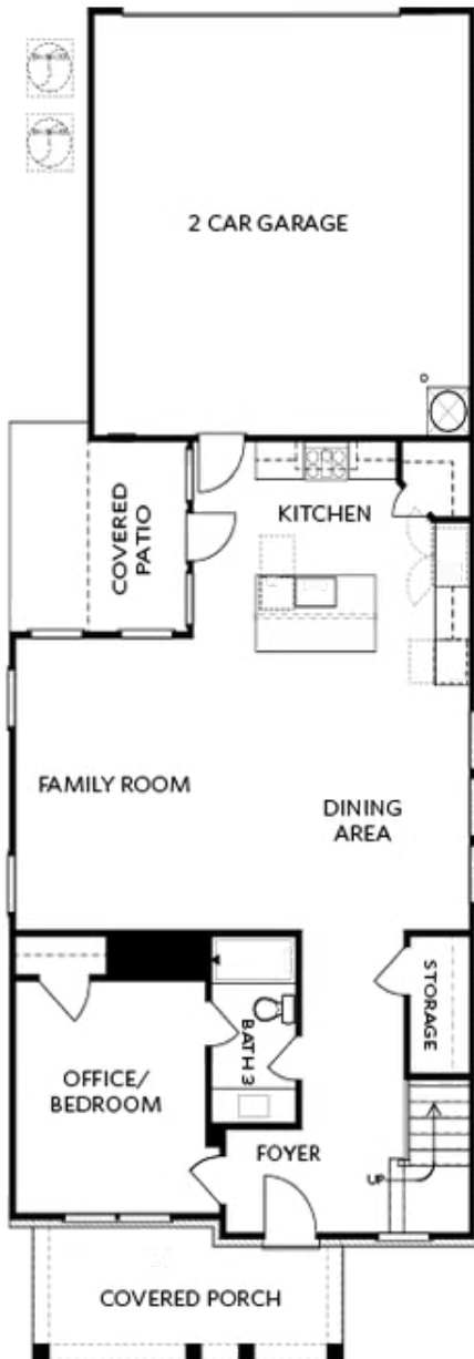
Elevation B
