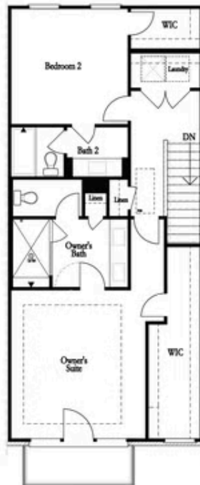
Elevation O
